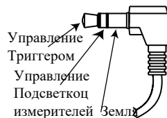
Рисунок 06— мини-штекер управления питанием
