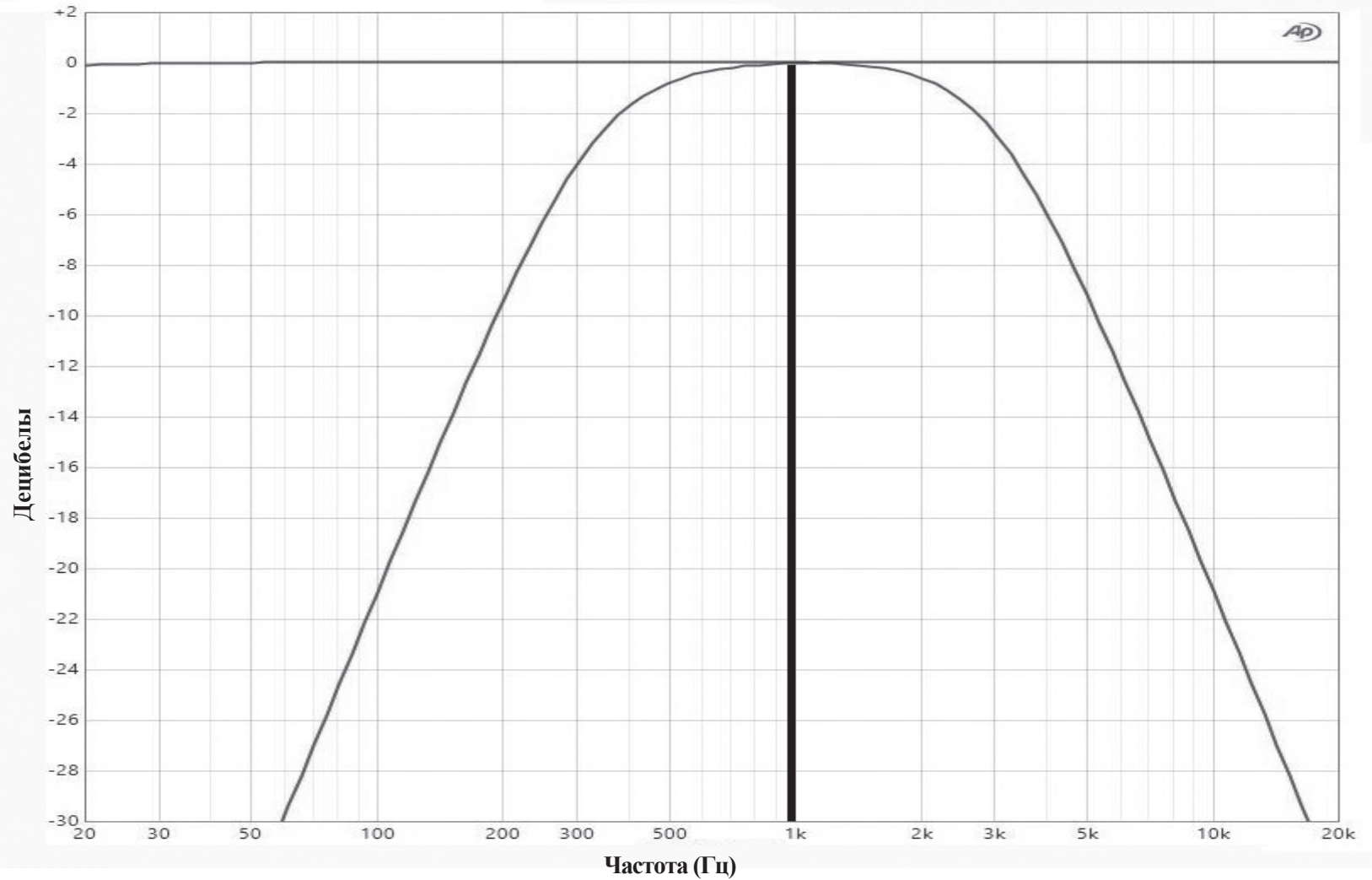
Рисунок 20– Комбинированный график спада 1K
