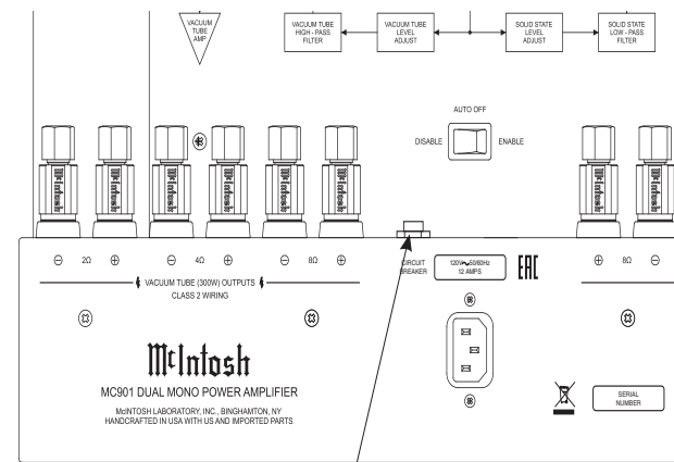
Рисунок 12— Автоматический размыкатель
