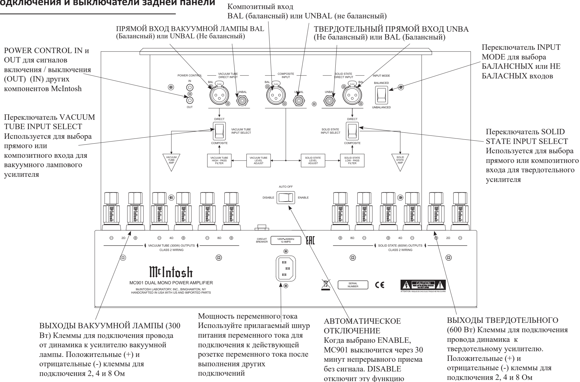
Рисунок 04- Вид сзади
