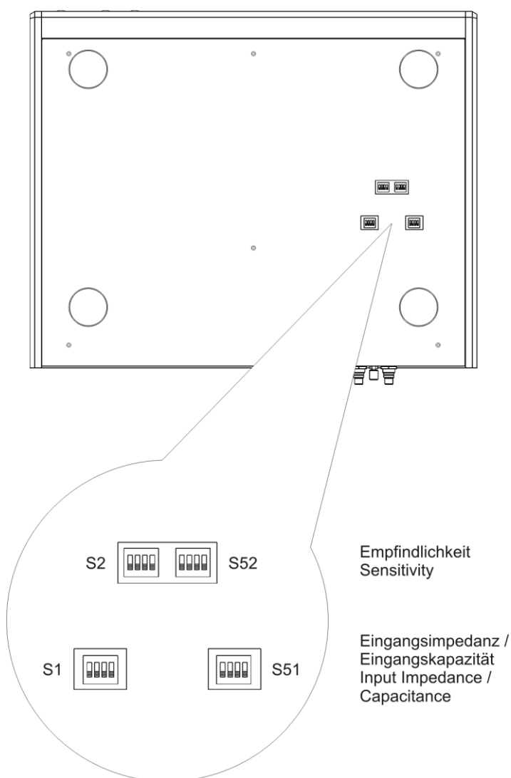
Abb.1: G 2000 R Ansicht von unten
