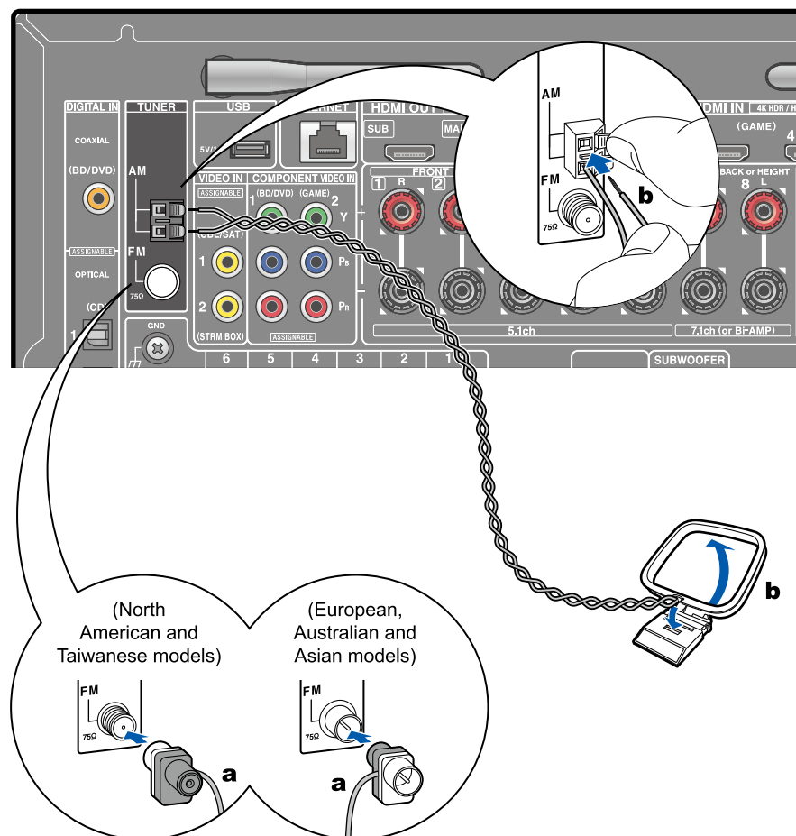
a Комнатная FM антенна, b Рамочная AM антенна
