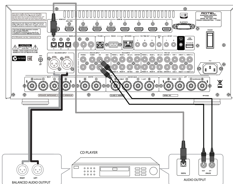
Cd-speleraansluitingen Collegamento di un lettore CD CD-spelare Подключения CD-плеера
