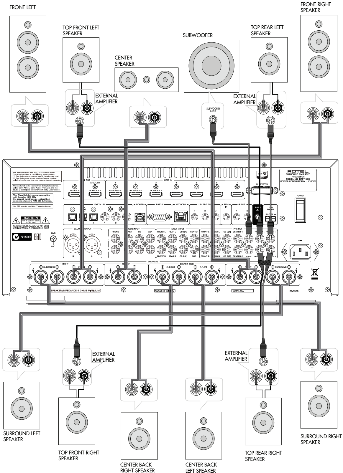
Figure 4: Speaker Connection Connexion de haut-parleur Lautsprecheranschluss Conexión de los altavoces
