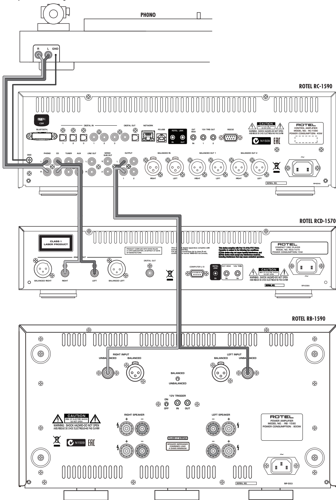
Analoge ingangen en utgangen Collegamenti ingressi ed uscite analogici Anslutningar för analoga in- och utgångar Аналоговые входы и выходы
