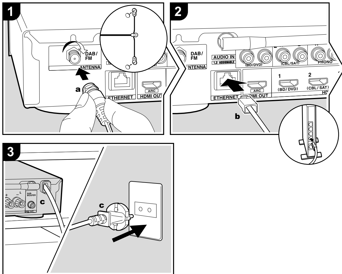
a Антенна DAB/FM, b Кабель Ethernet, c Кабель питания.
