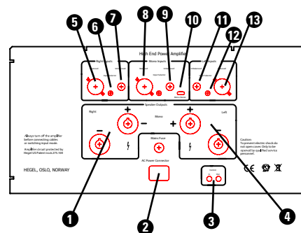
Задняя панель H30
