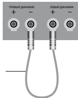
Закорачивающая перемычка
